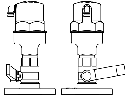
S-050 TAP&FLANGE DN25
